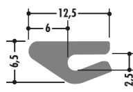
Hava Konveyör Profili
