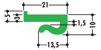
Geçmeli Z Profili
